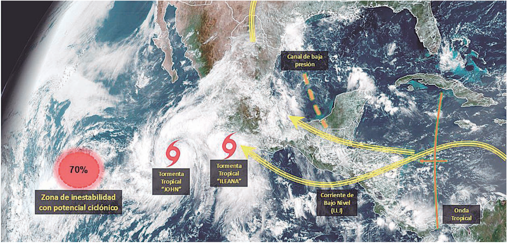
Imagen del Servicio Meteorológico Nacional
